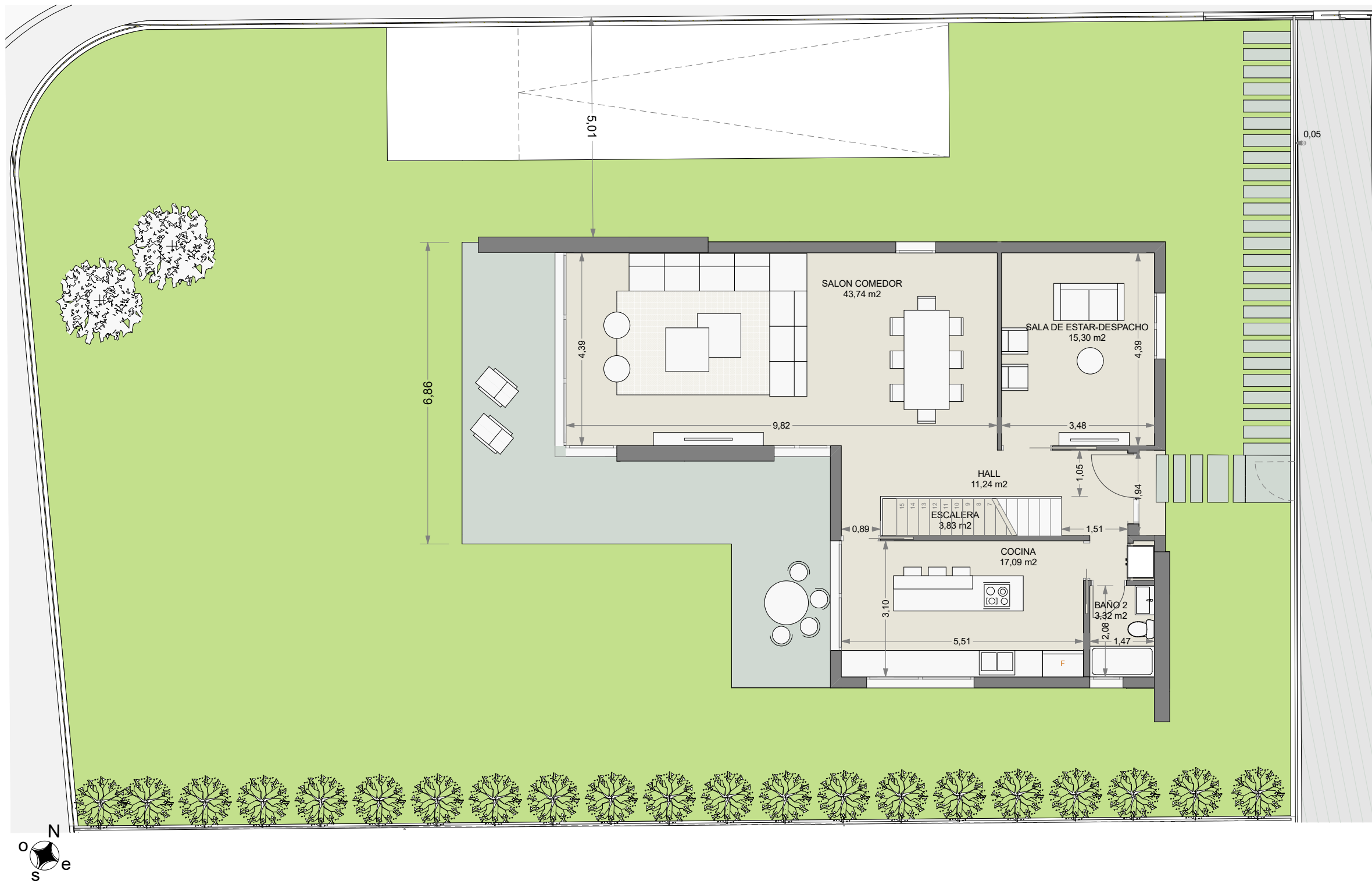
PARCELA 01. TIPOLOGÍA 2. Escala 1/100
